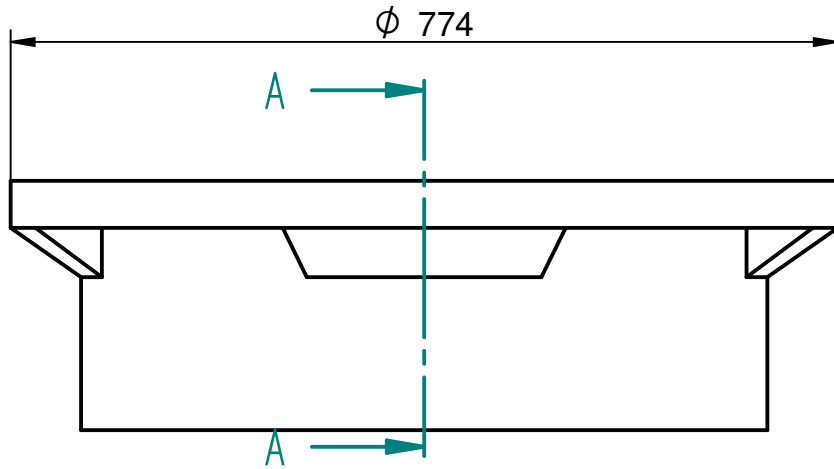
Schnitt A-A
